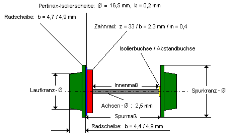
Maßbezeichnungen Radsatz BR 42
