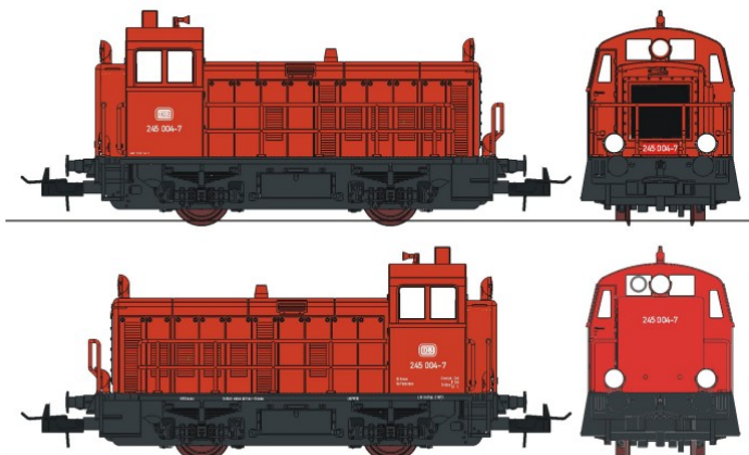
BR 245 Aufriss
